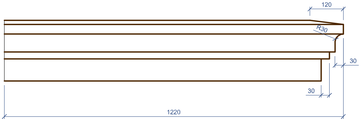
Вид слева (Масштаб 1:2)
