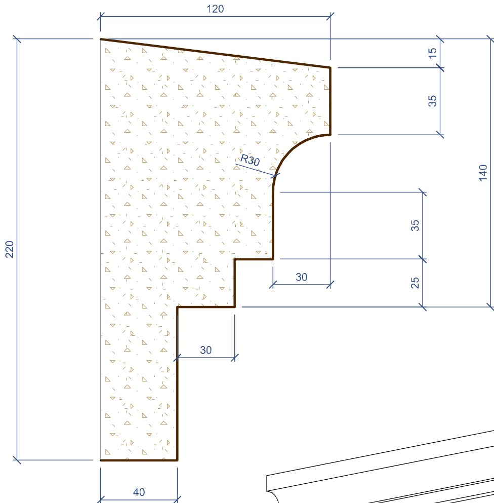
Вид слева (Масштаб 1:2)
