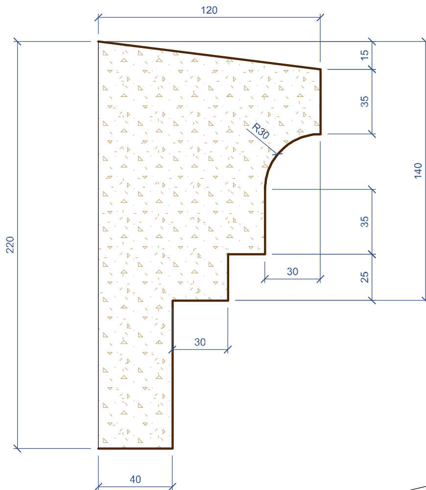
Вид слева (Масштаб 1:2)
